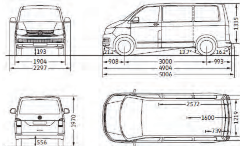
Caravelle 短軸版 尺寸圖
