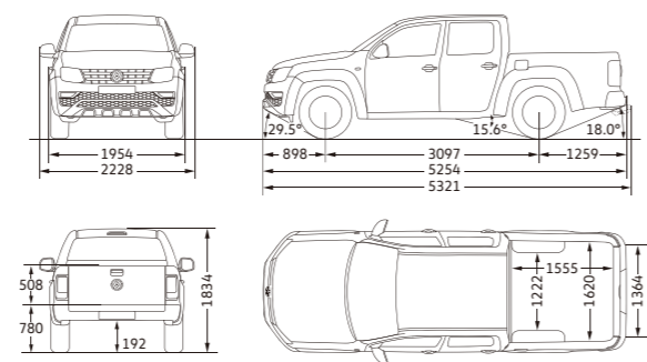
Amarok V6 尺寸圖
